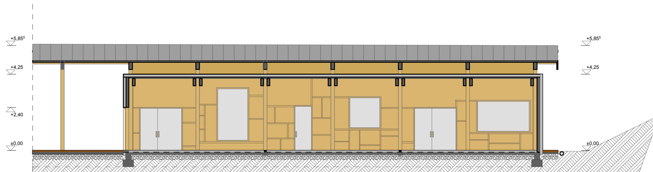
A4-A4 METSZET
