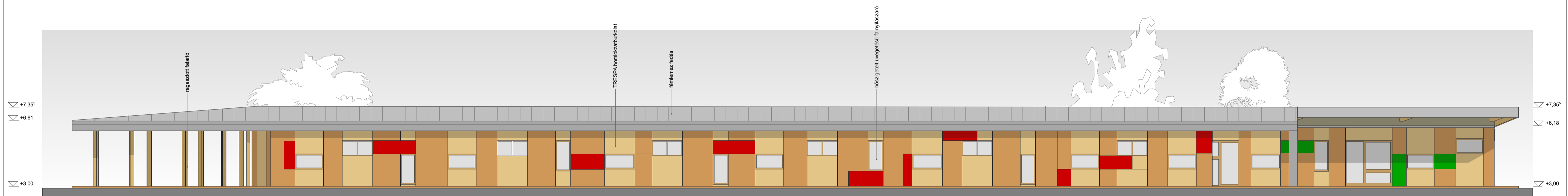
"B" HOMLOKZAT É-K I. m= 1:100
