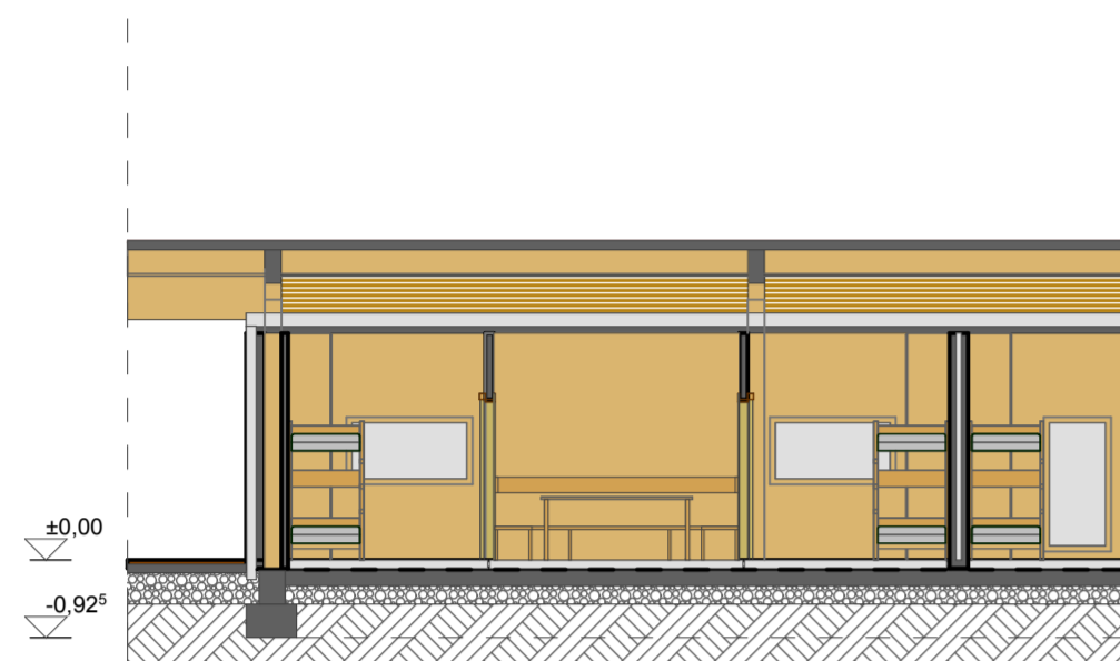
B2 METSZET
