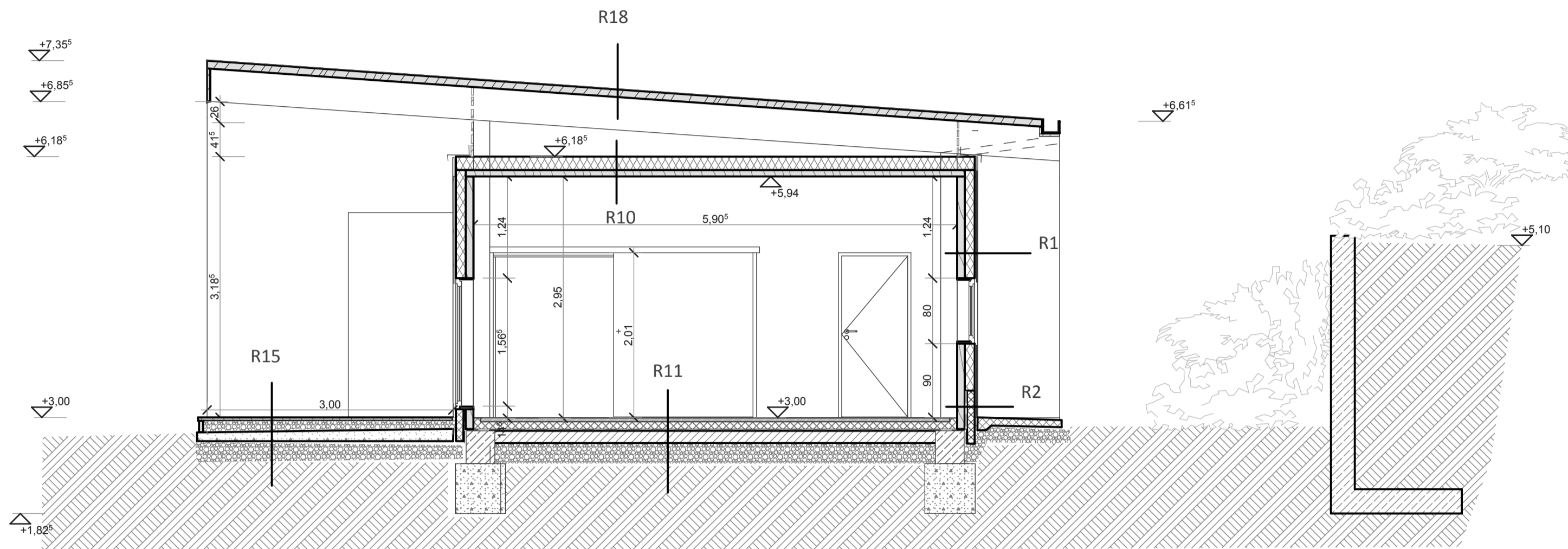
B-B METSZET M= 1:50
