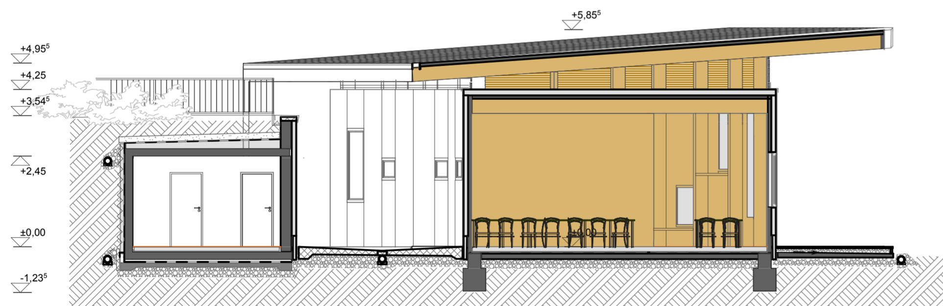
A2-A2 METSZET
