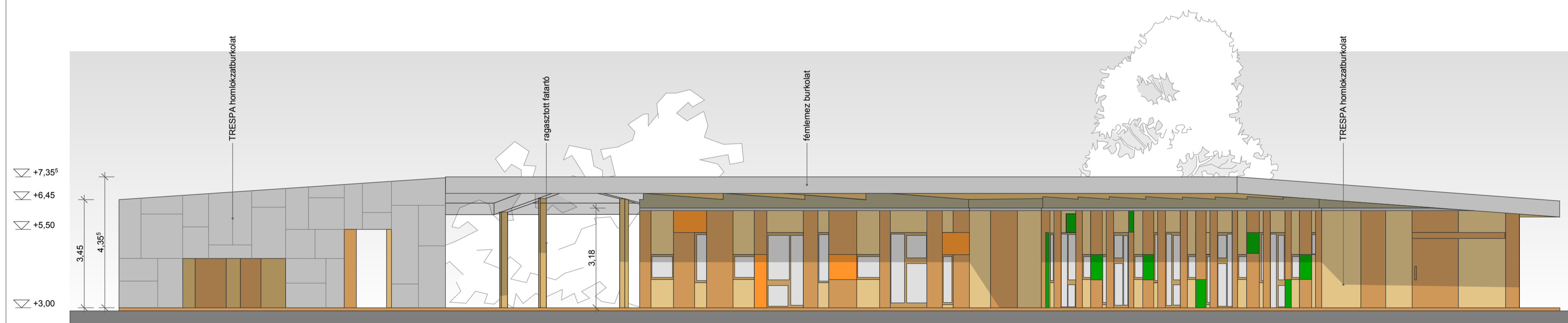
"B" HOMLOKZAT D-K m= 1:100
