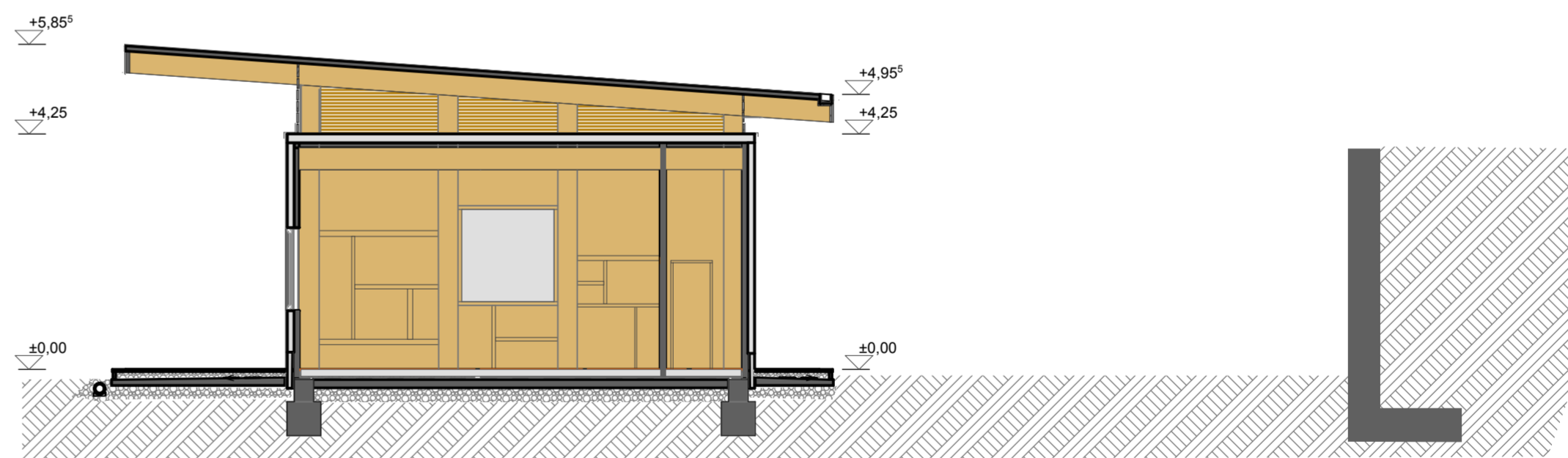
A3-A3 METSZET
