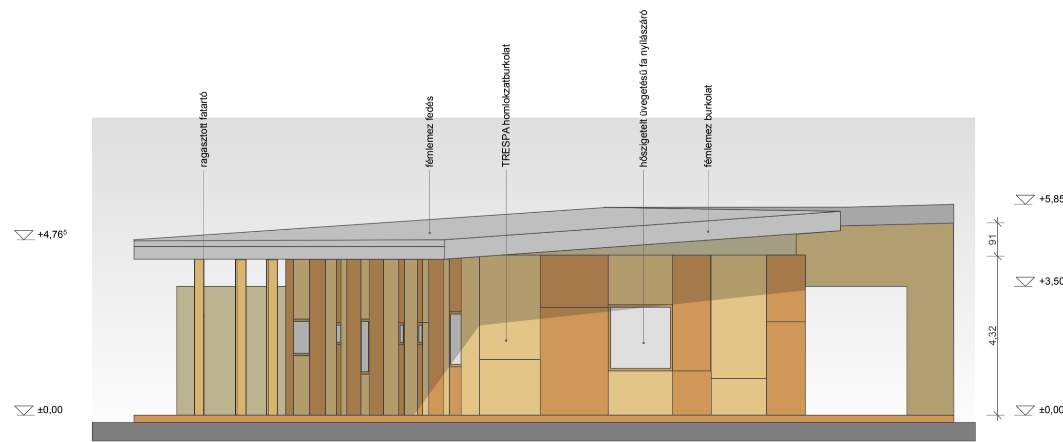
"A" HOMLOKZAT D-Km= 1:100
