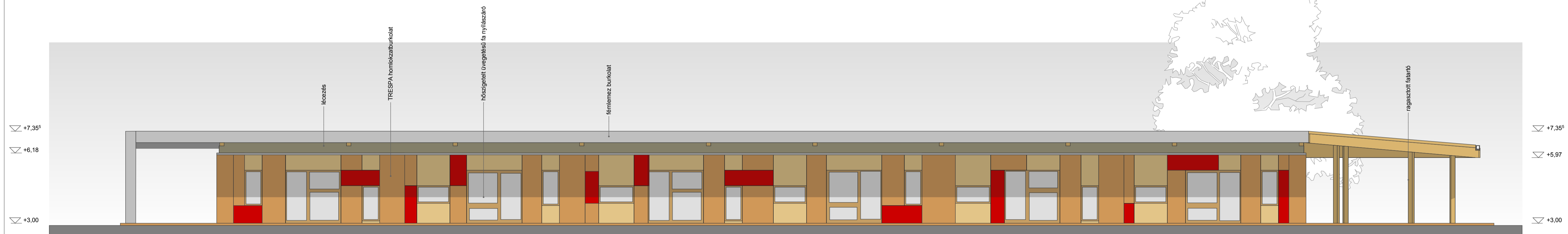
"B" HOMLOKZAT D-K I. m= 1:100
