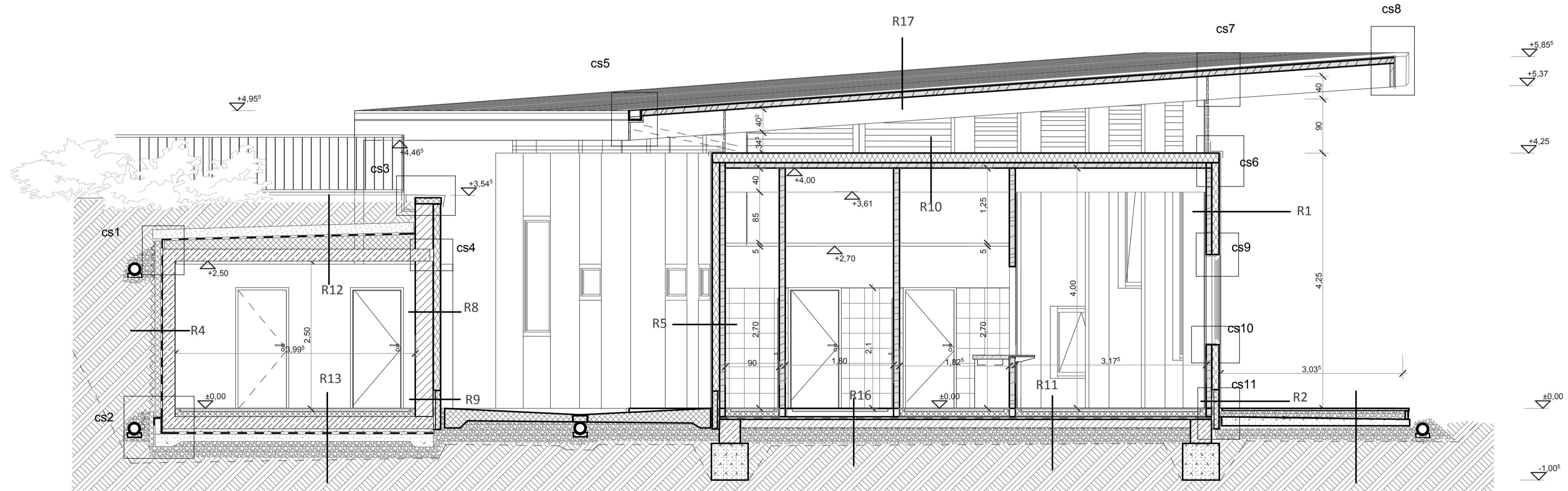
A-A METSZET M= 1:50
