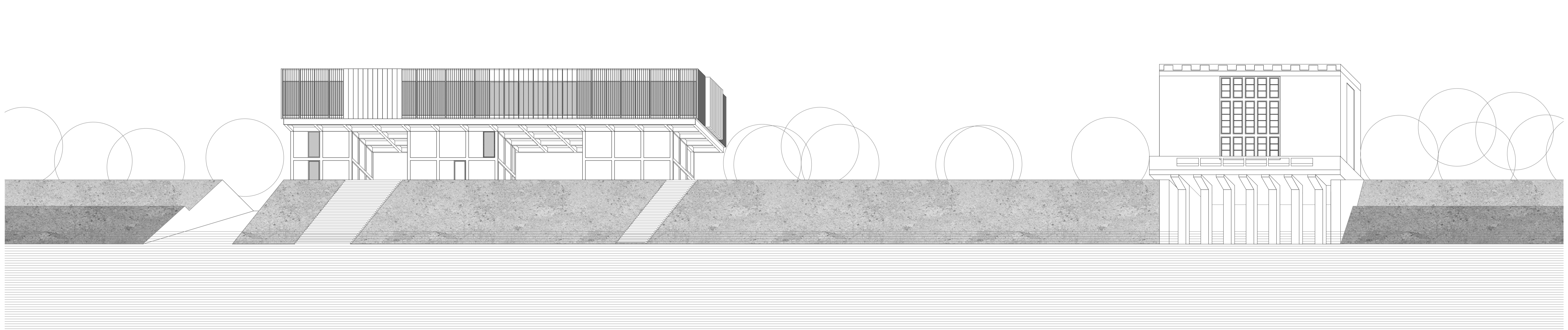
TISZA PARTI HOMLOKZATOK M1/200
