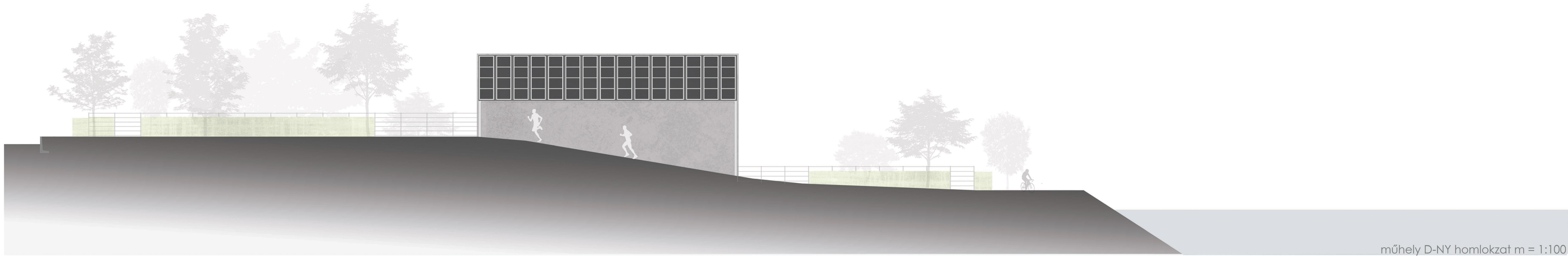
műhely D-NY homlokzat m = 1:100
