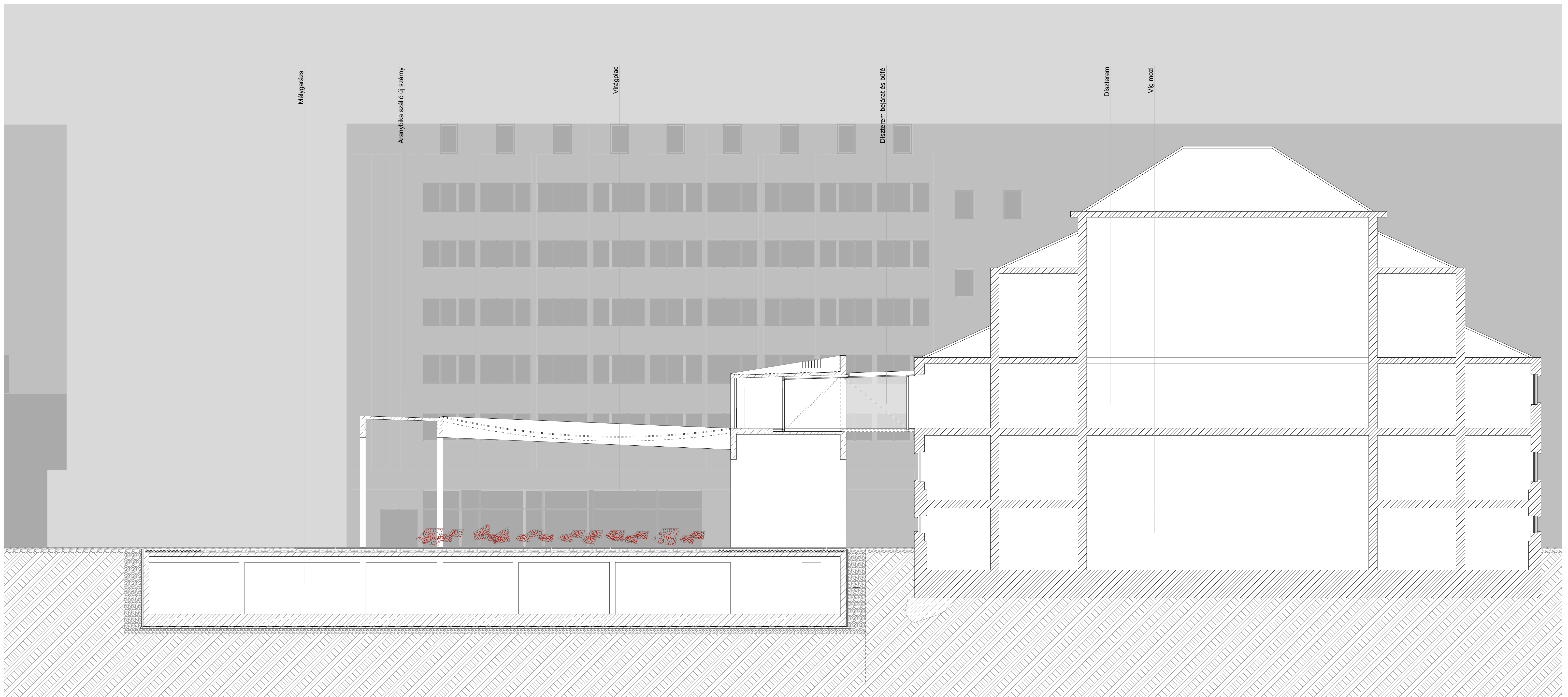
Keresztmetszet, Aranybika szálló felé, M=1:100
