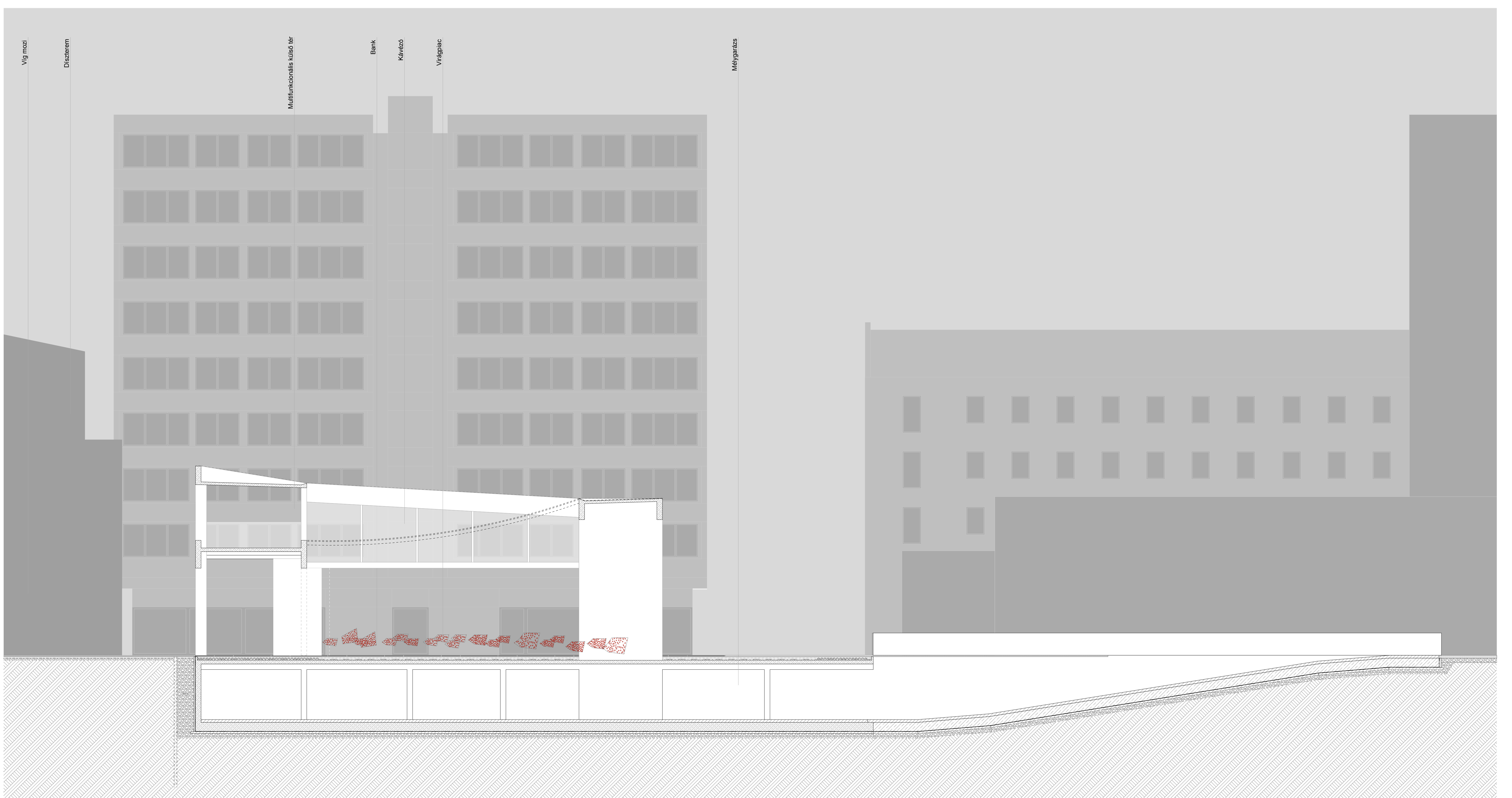
Keresztmetszet, Tömbbelső felé, M=1:100
