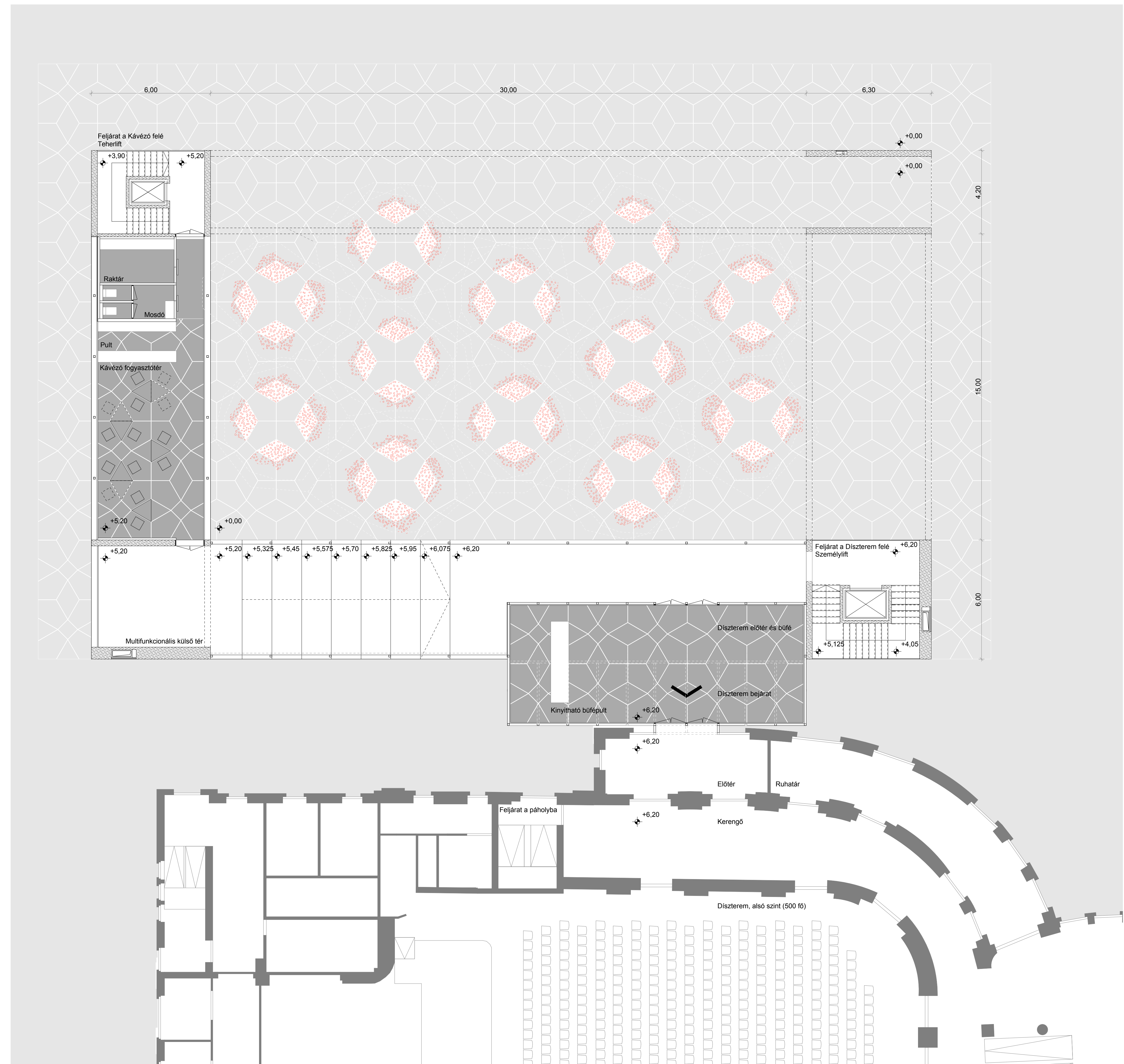
Alaprajz, Emelet, M=1:100
