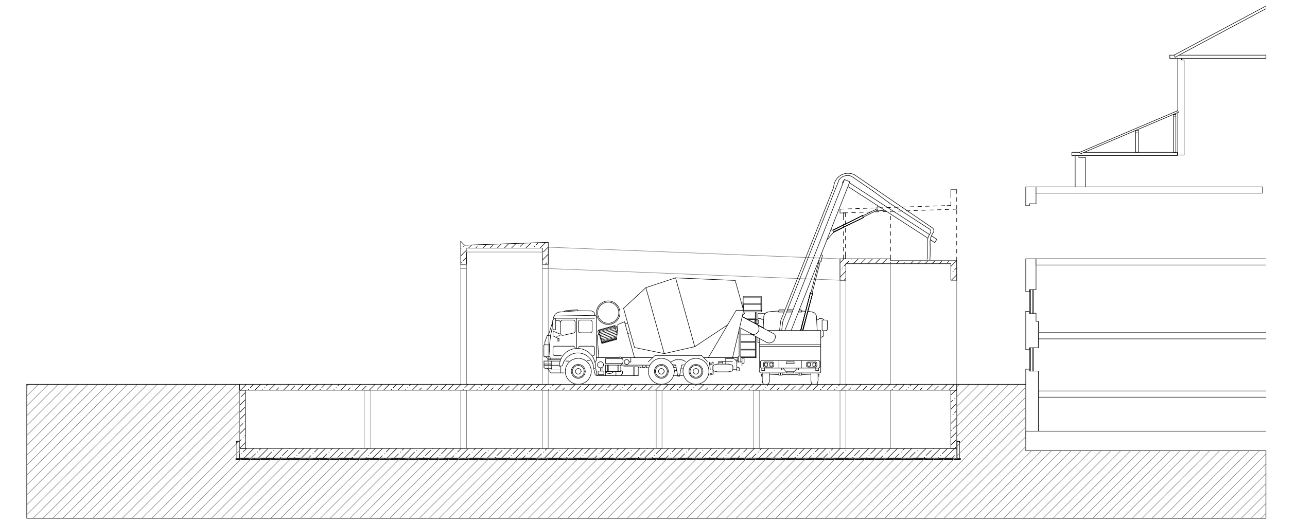
Metszet, szerkezetépítési fázis, M=1:200
