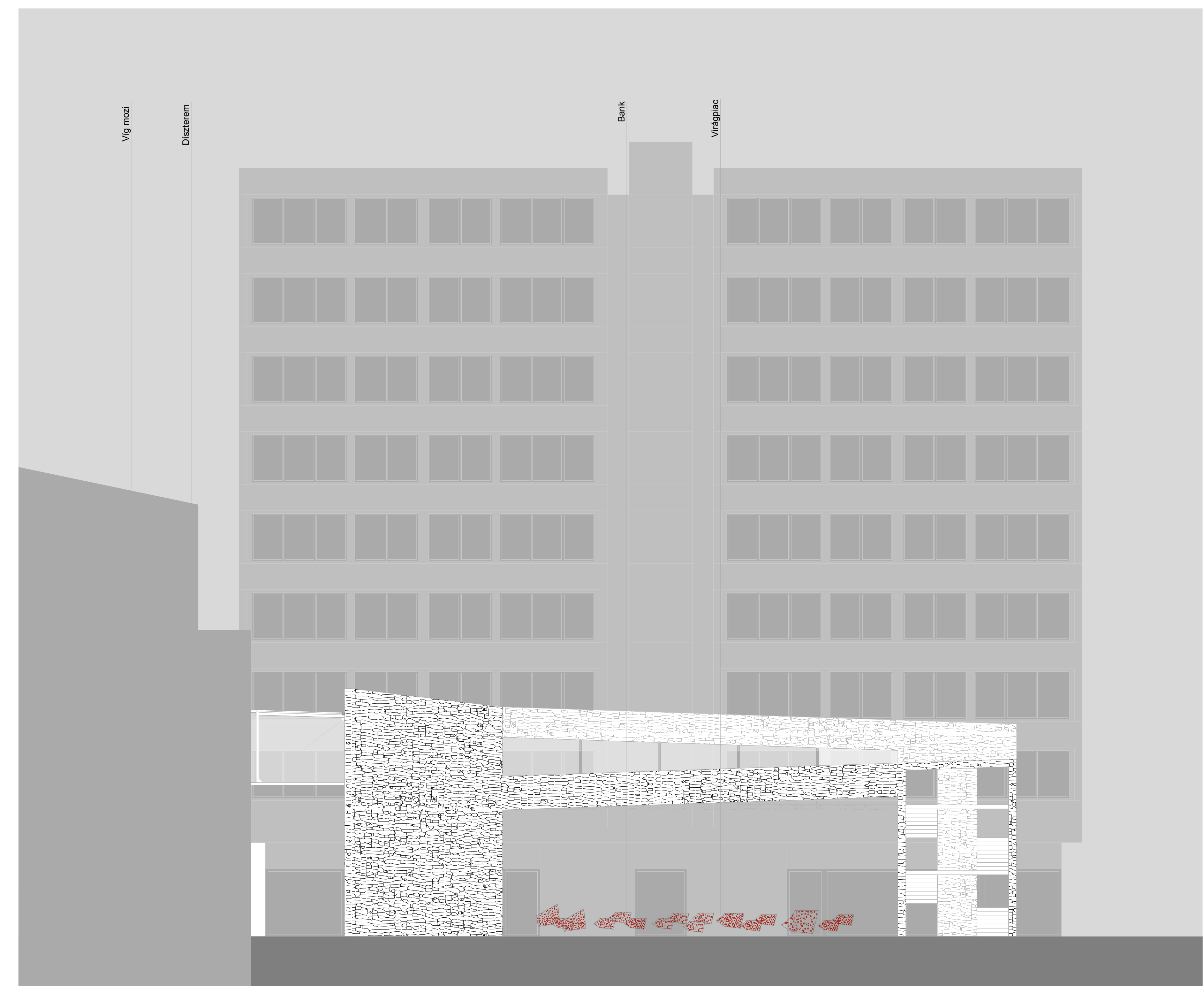
Homlokzat, Tömbbelső felé, M=1:100
