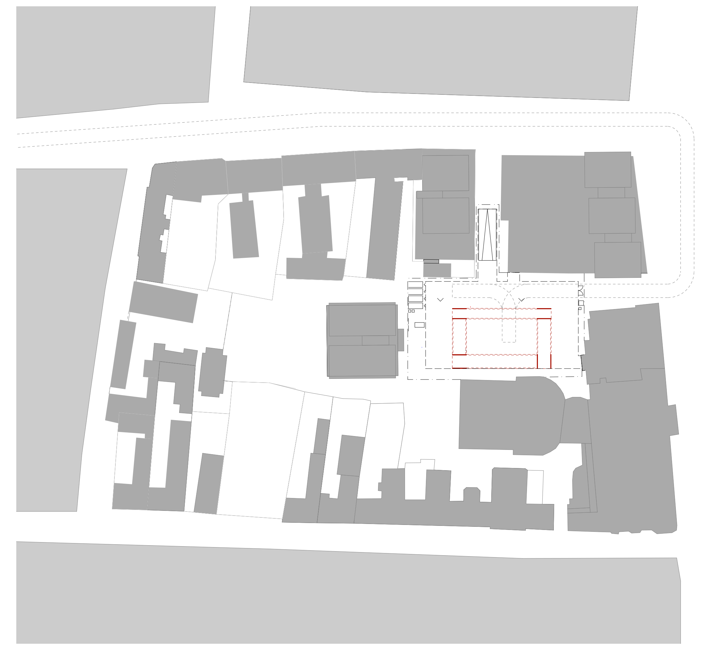
Organizációs helyszínrajz, szerkezetépítési fázis, M=1:1000
