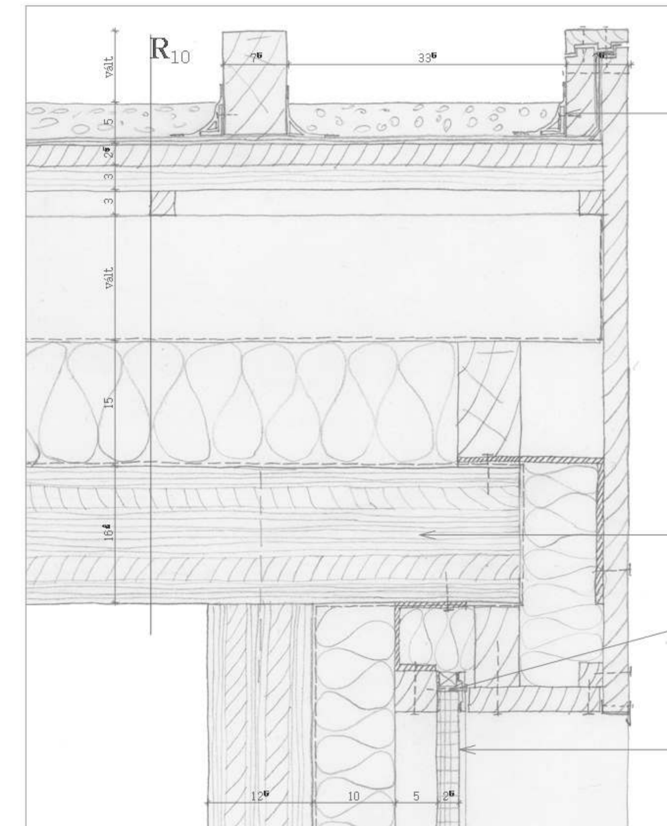
CS10 F – TETŐ OROMZATI KIALAKÍTÁSA FÖDÉM ÉS POLIKARBONÁT BURKOLAT FELSŐ CSATLAKOZÁSA
