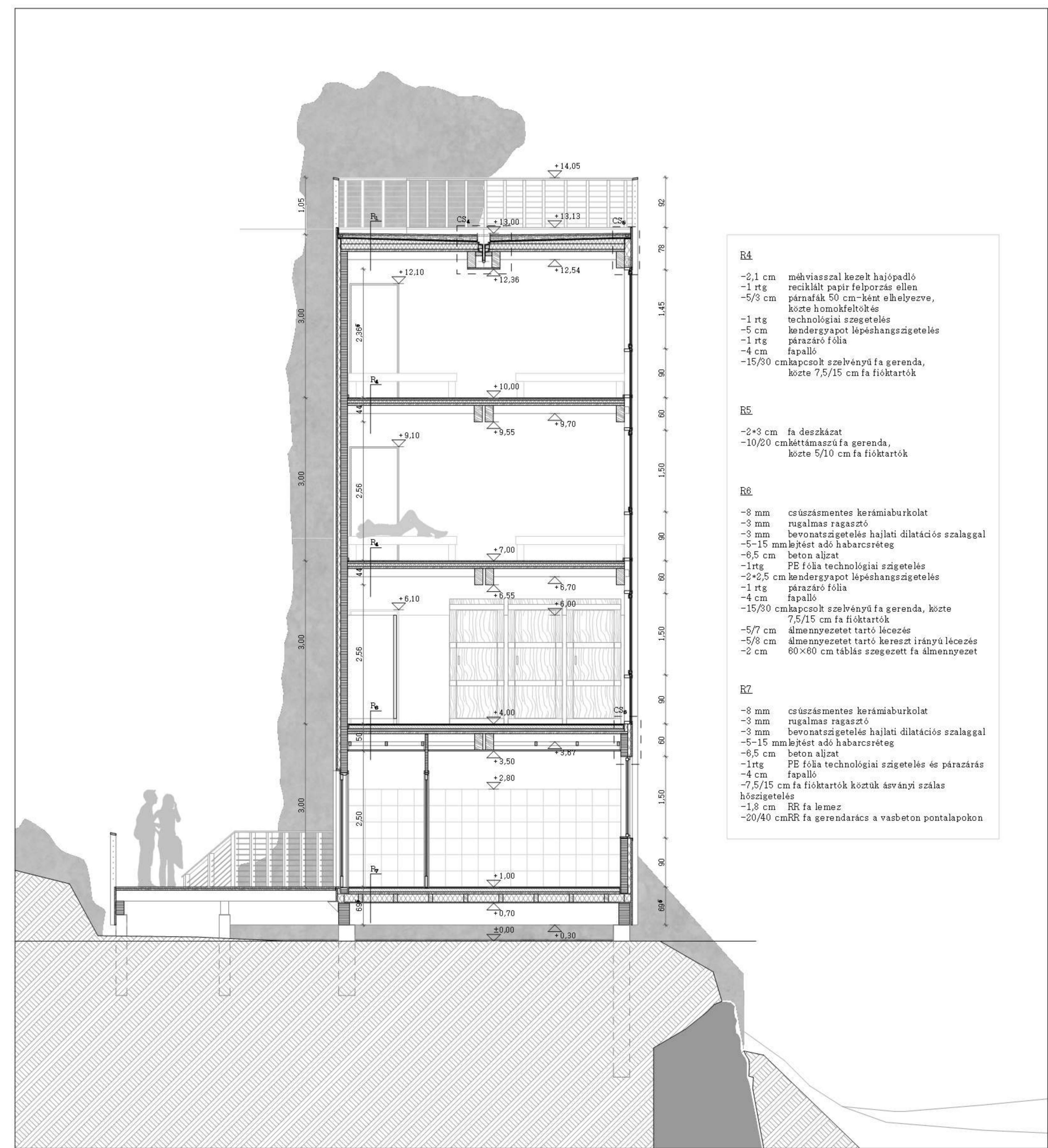
D-D METSZET
