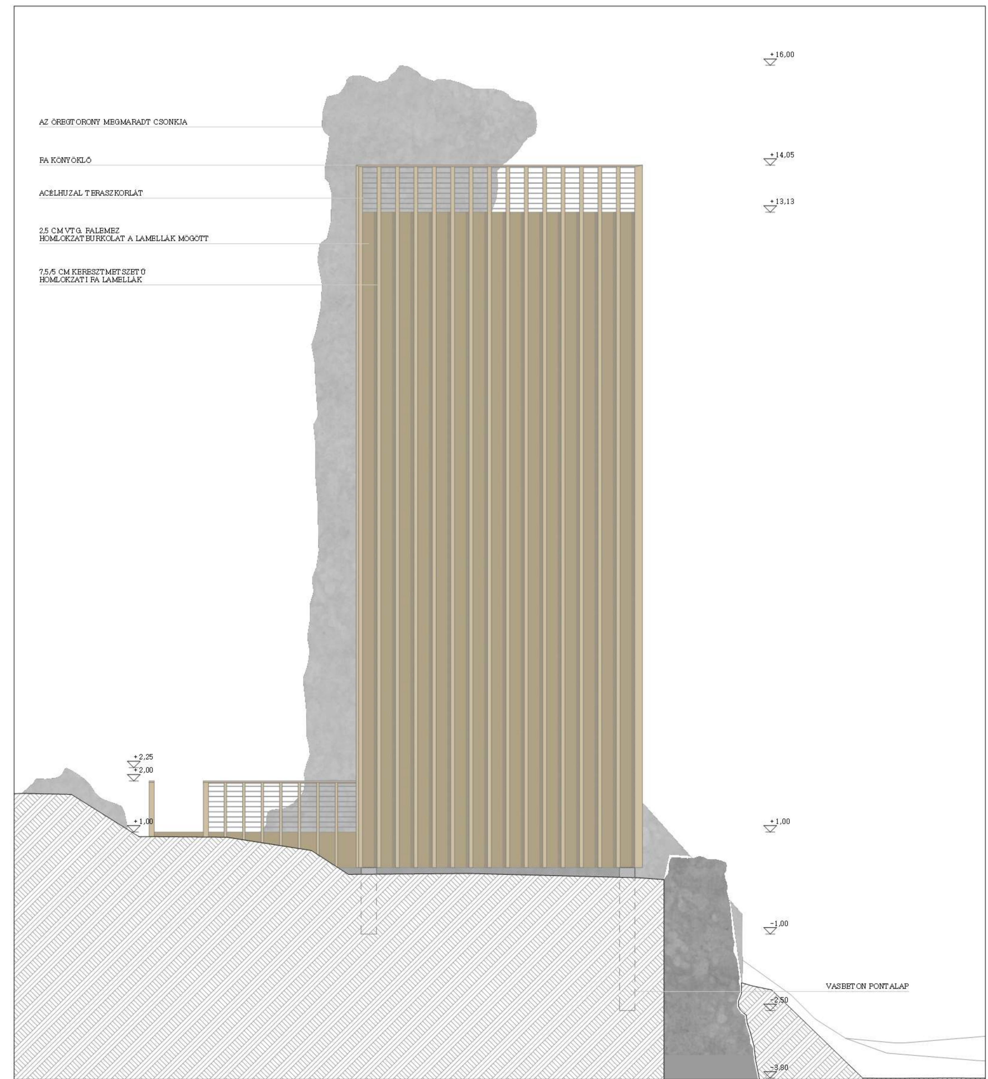
ÉSZAKKELETI HOMLOKZAT
