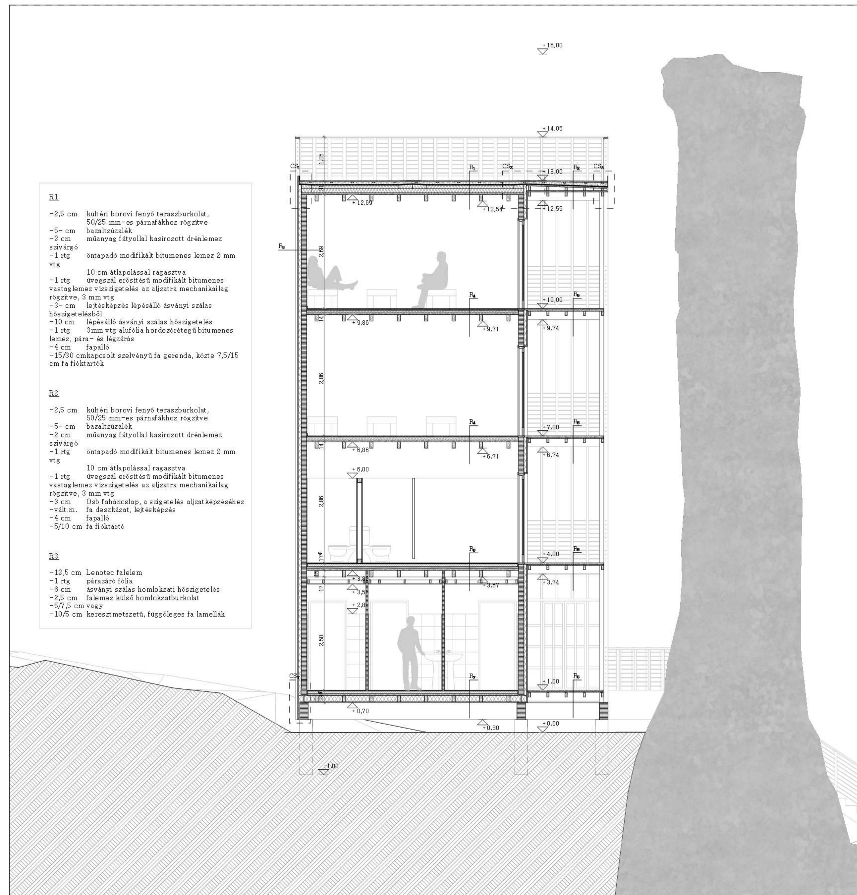
C-C METSZET
