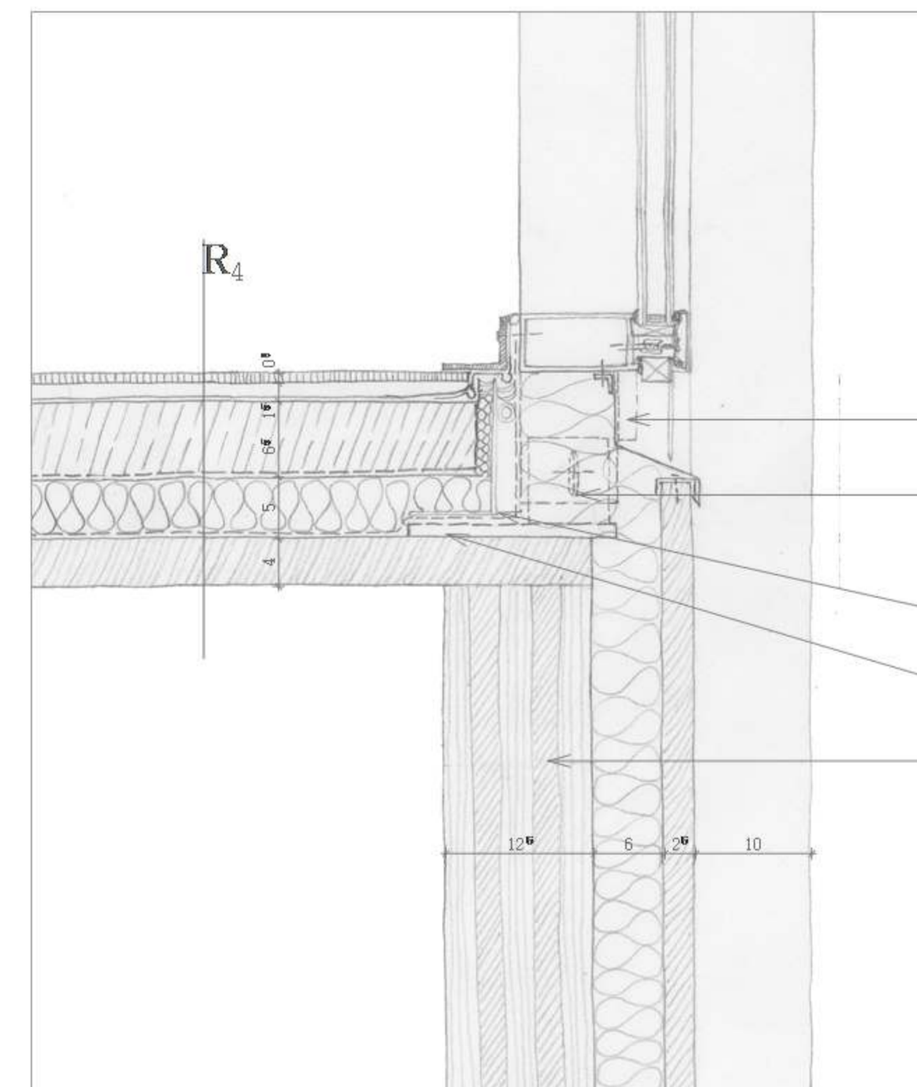
CS6 T – HOMLOKZATI BURKOLATVÁLTÁS
