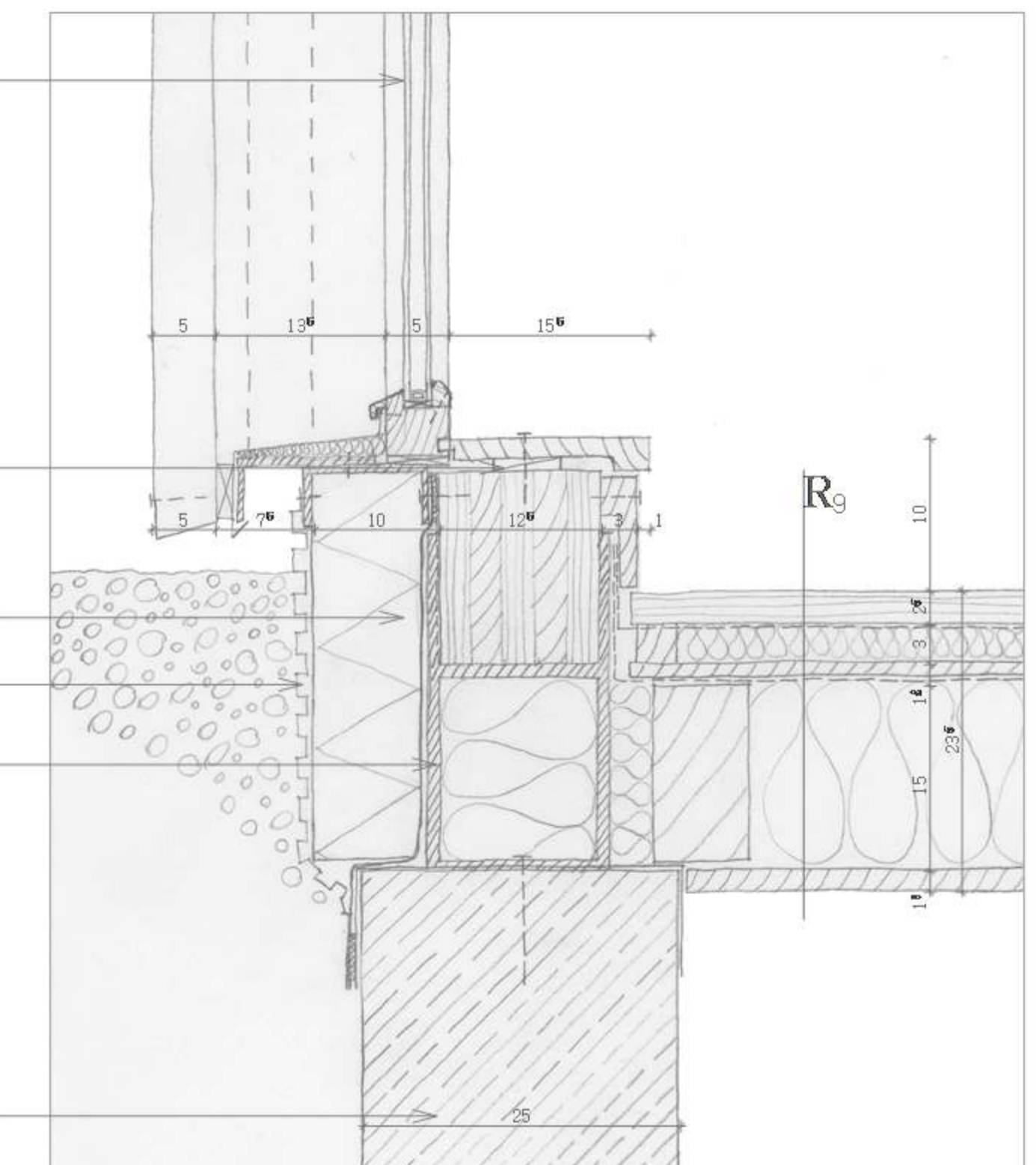
CS13 F – LÁBAZATI KIALAKÍTÁS A VÁRDOMB FELŐLI OLDALON
