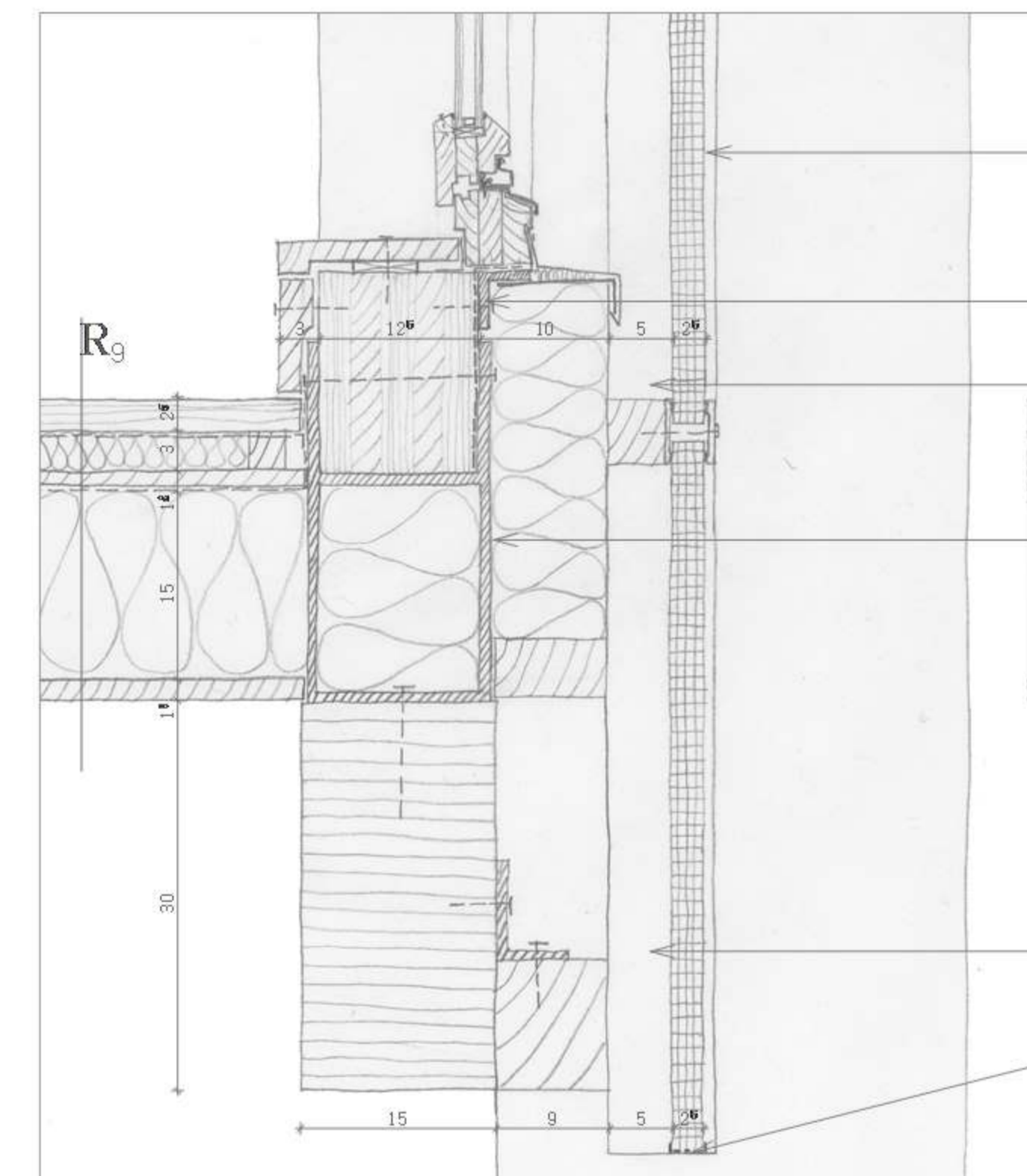
CS11 F – POLIKARBONÁT HOMLOKZATI BURKOLAT ALSÓ LEZÁRÁSA
