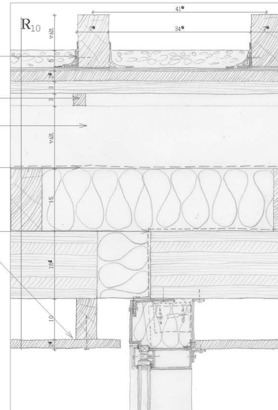
CS9 F – FEDETT TERASZNÁL FÖDÉM ÉS FÜGGŐNYFAL ALSÓ CSATLAKOZÁSA
