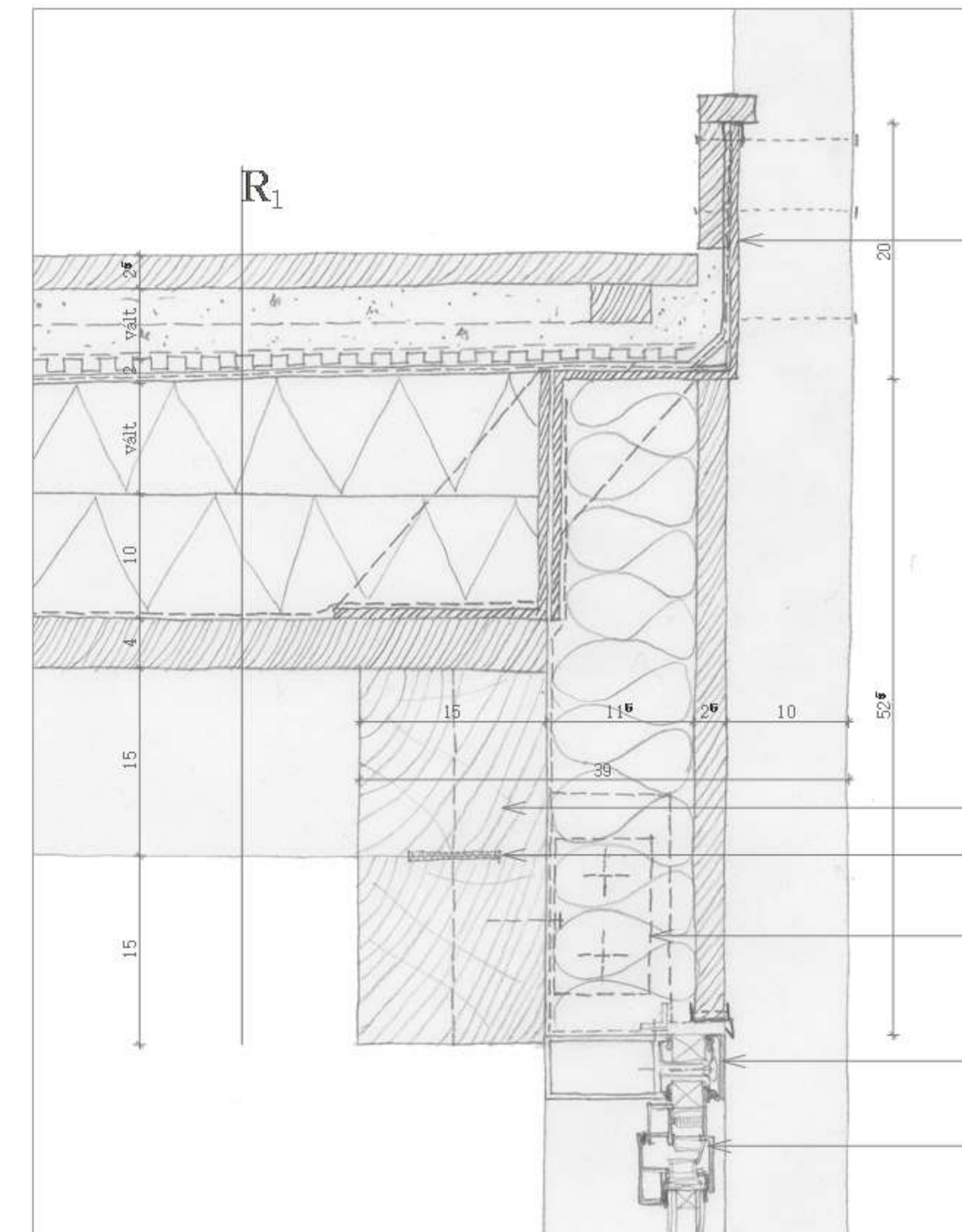
CS5 T – TETŐTERASZ "ATTIKAKIALAKÍTÁS" HOMLOKZATI BURKOLATVÁLTÁS
