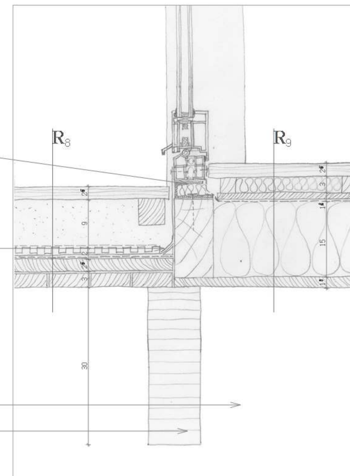
CS9 F – FEDETT TERASZNÁL FÖDÉM ÉS FÜGGŐNYFAL ALSÓ CSATLAKOZÁSA
