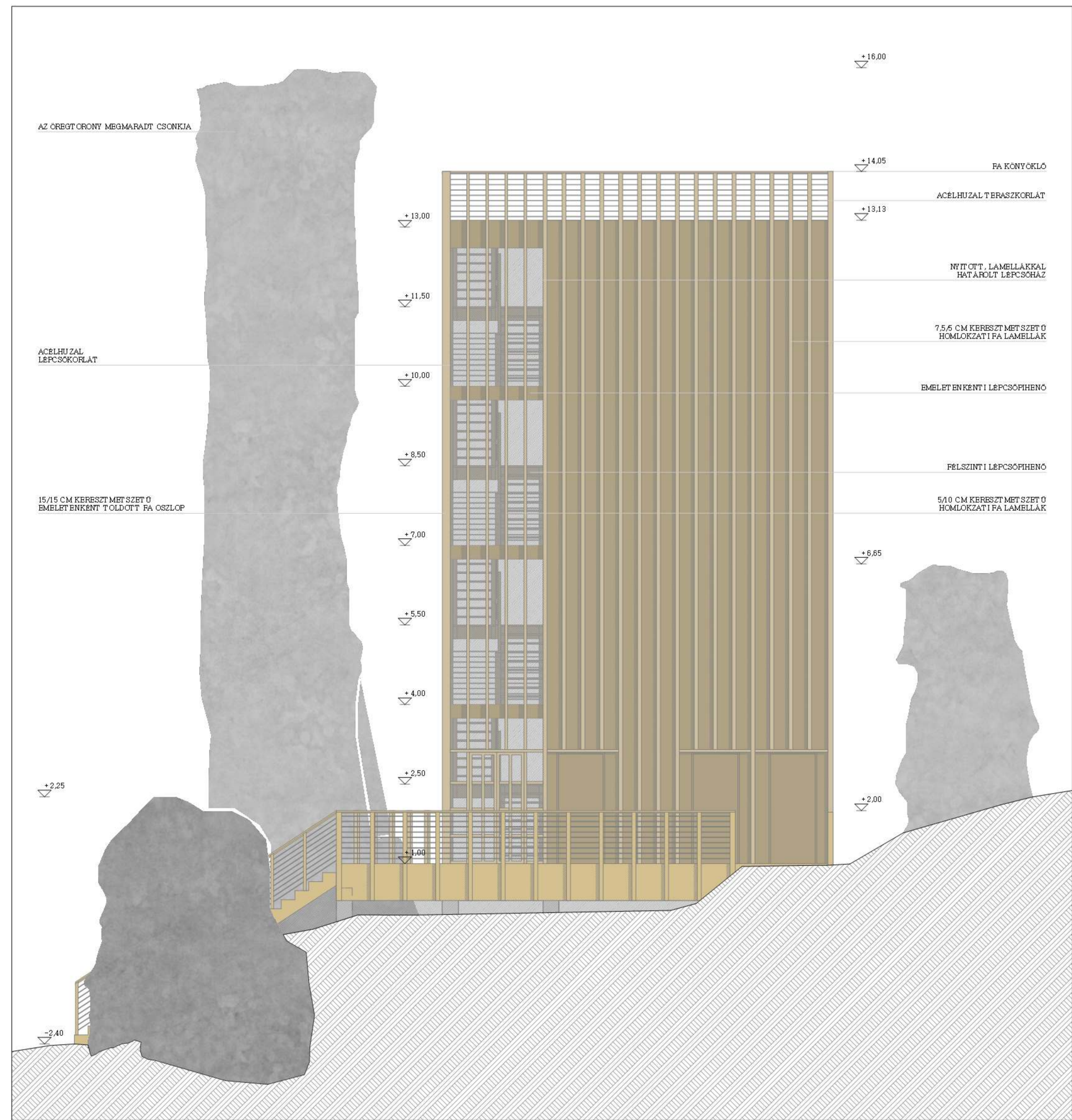
DÉLKELETI HOMLOKZAT
