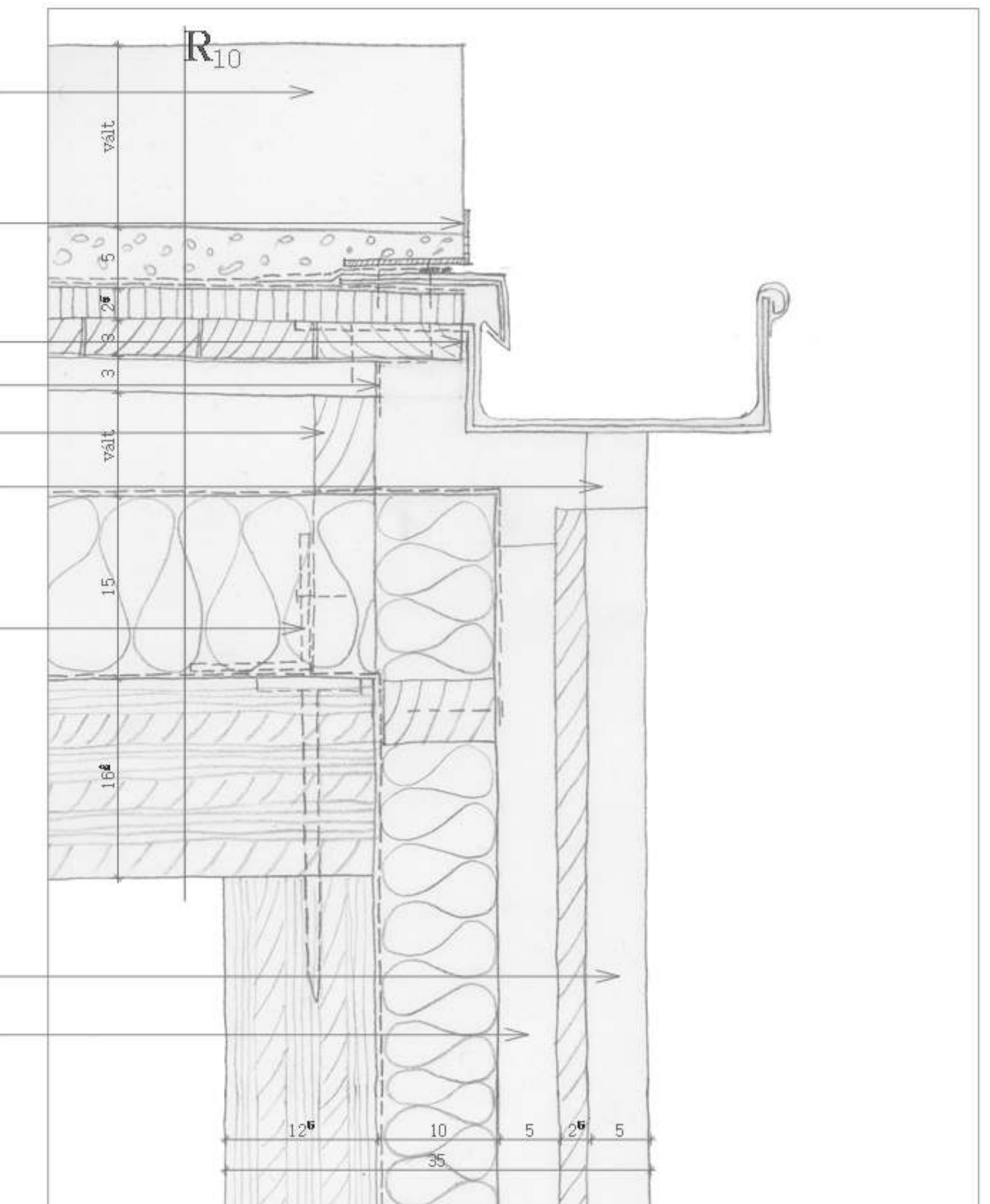
CS12 FOGADÓÉPÜLET ERESZKIALAKÍTÁSA
