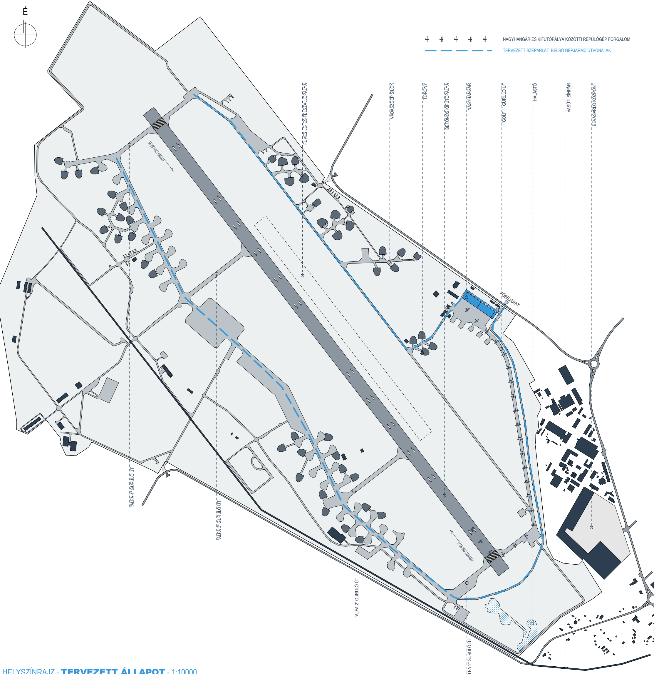
HELYSZÍNRAJZ - TERVEZETT ÁLLAPOT - 1:10000
