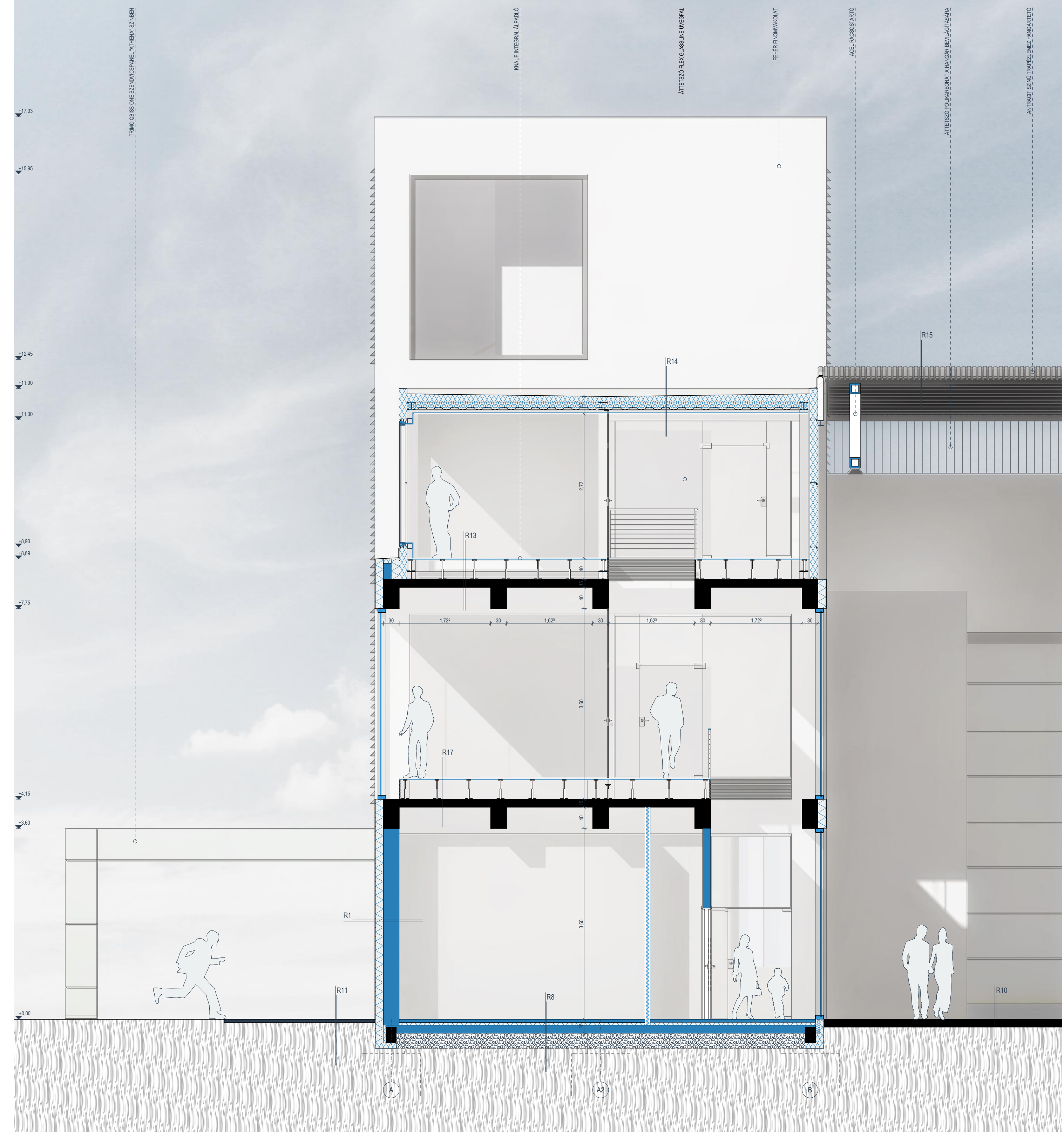
METSZET - C-C - M=1:50
