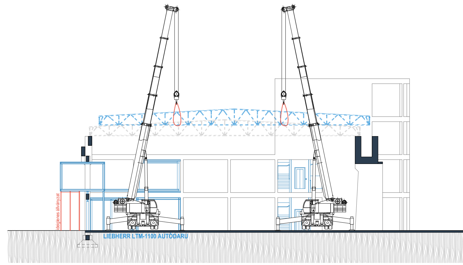
ORGANIZÁCIÓS METSZET - SZERKEZETÉPÍTÉS - M=1:250
