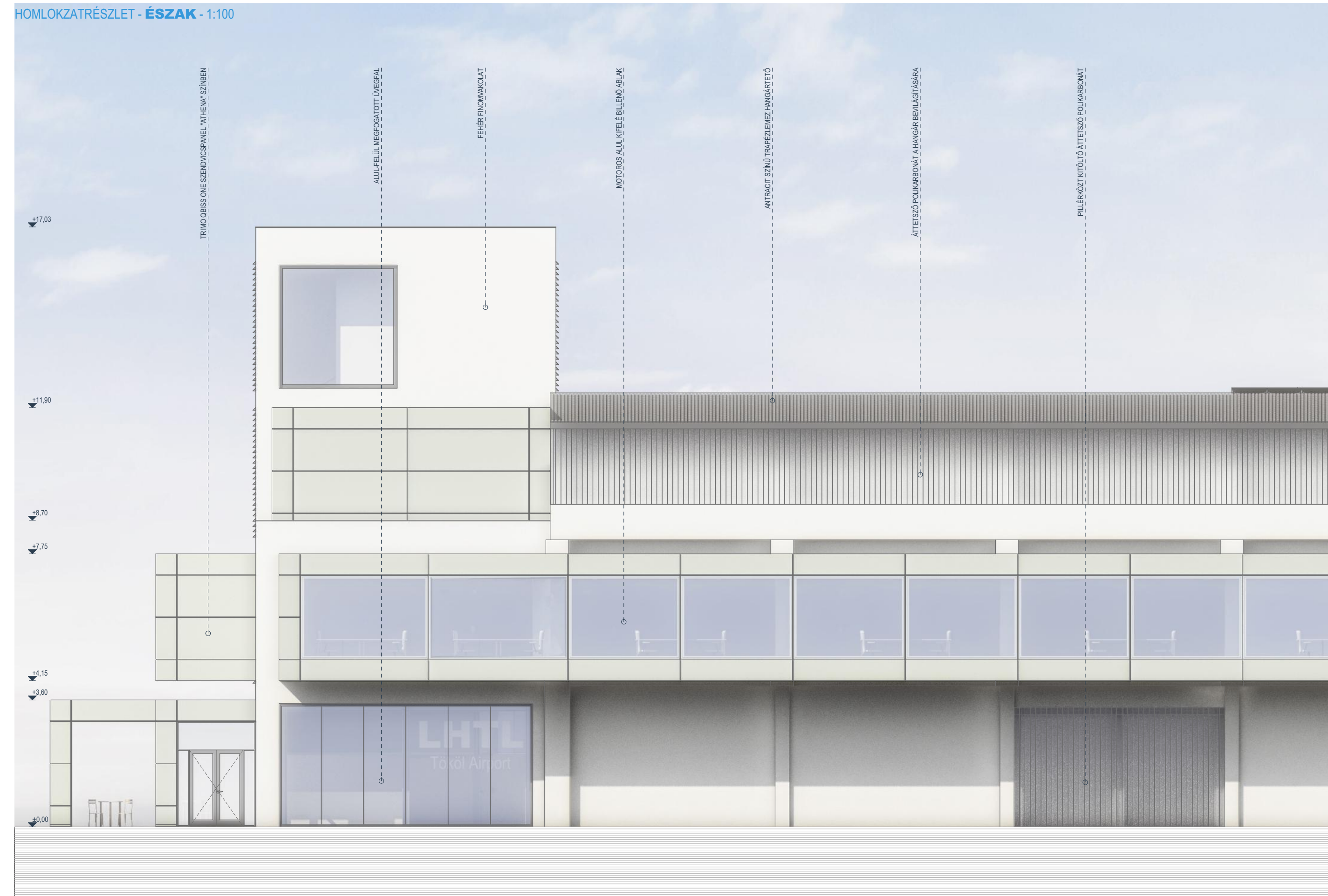
HOMLOKZATRÉSZELET - ÉSZAK - 1:100
