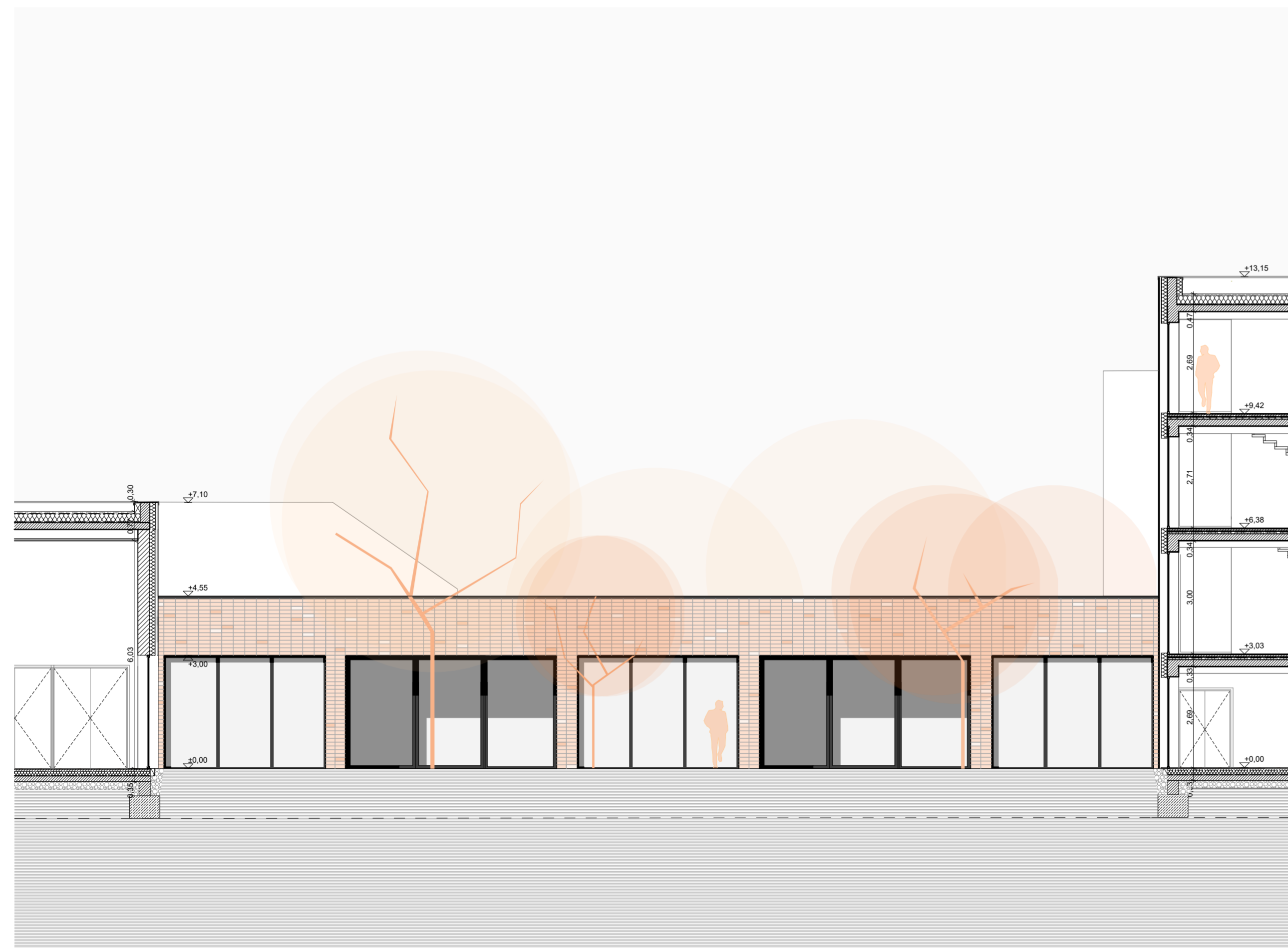
BELSŐ UDVAR HOMLOKZAT M=1:100
