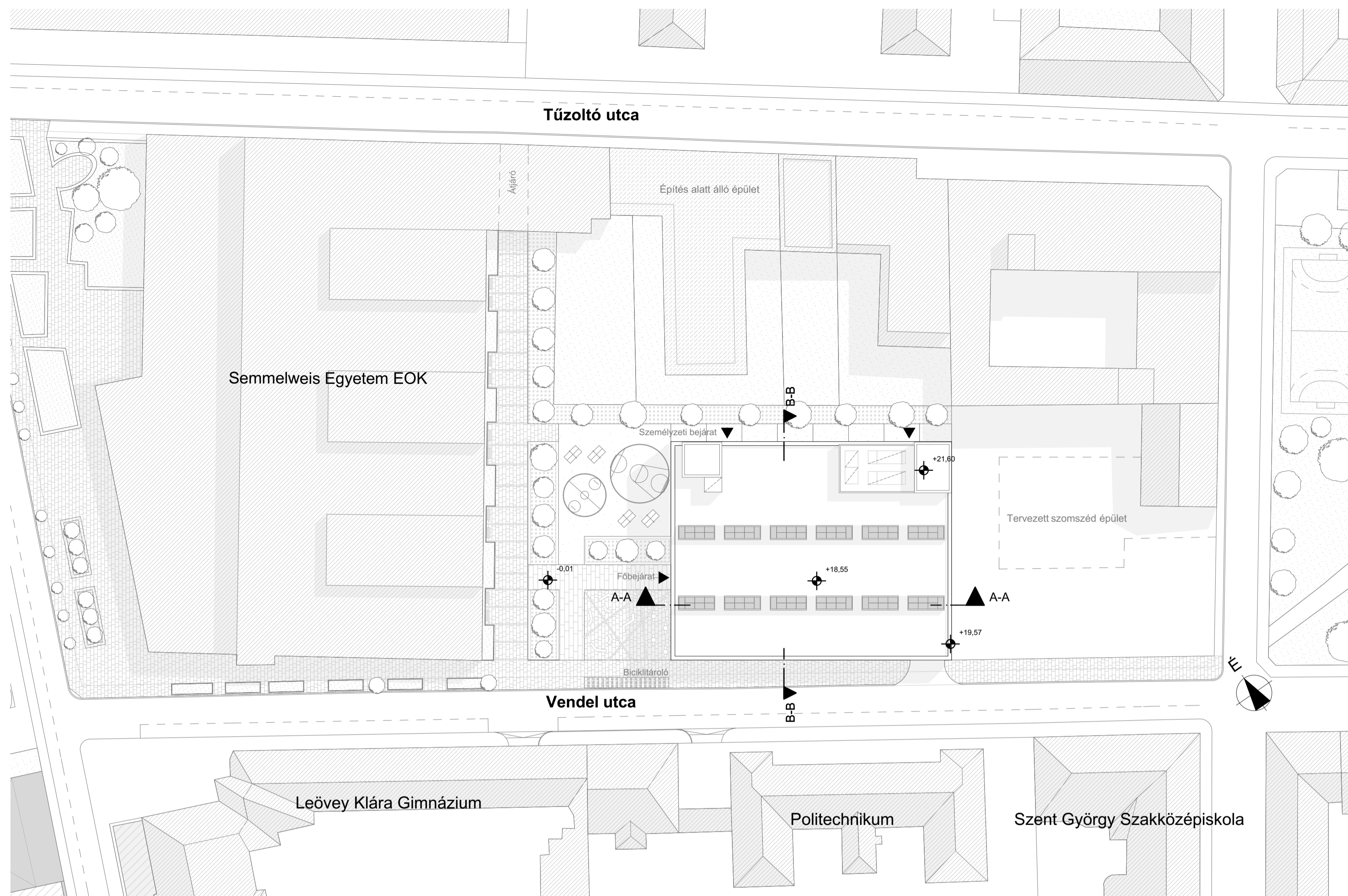
Helyszínrajz M=1:500
