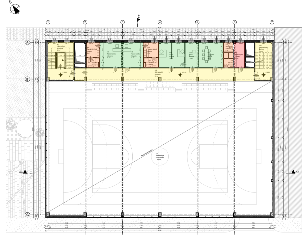
Funkcióséma M=1:400
