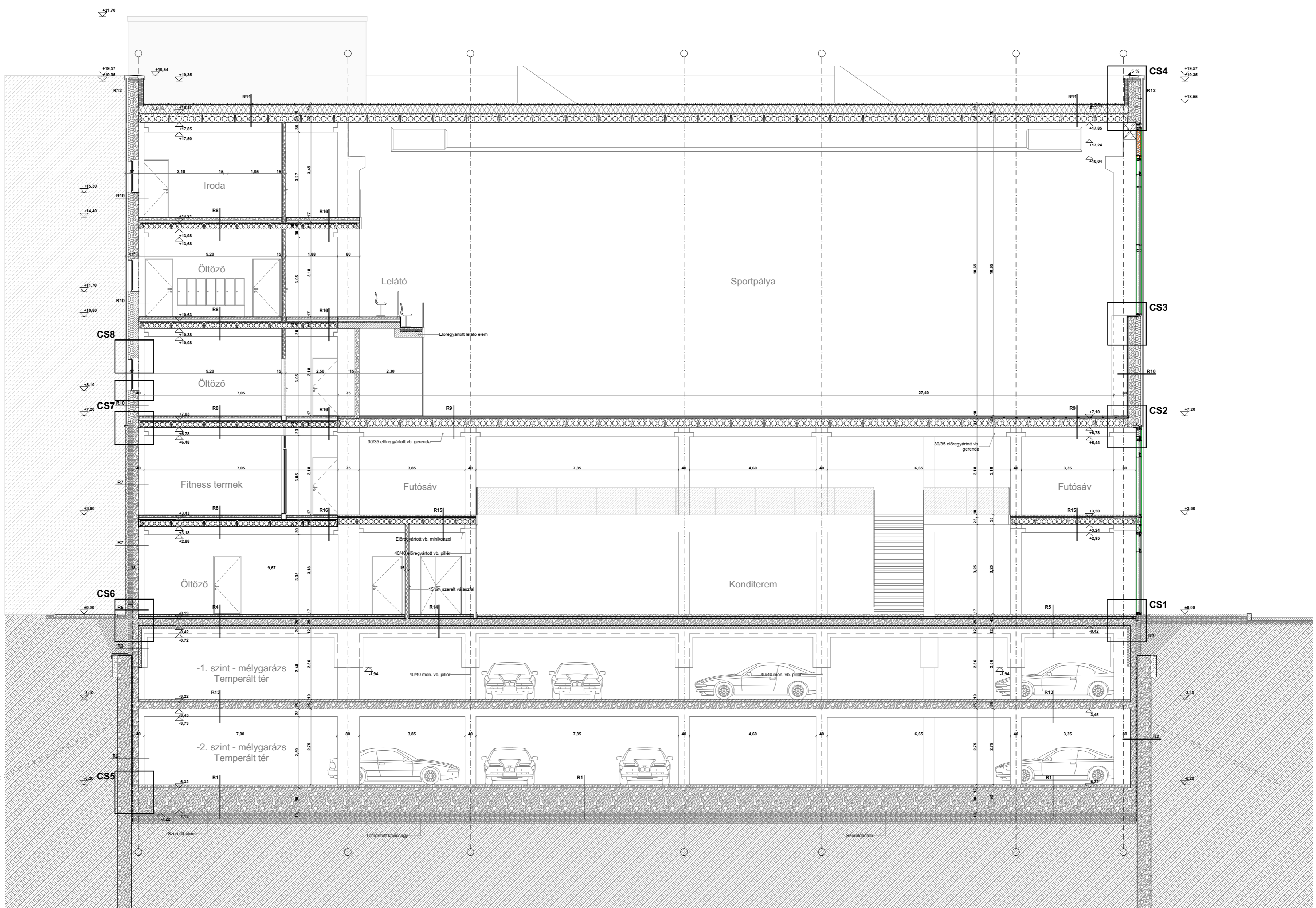
B-B metszet M= 1:100
