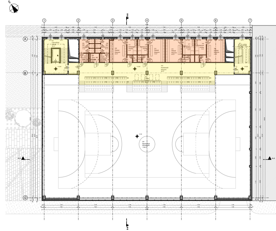
Funktionséma M=1:400
