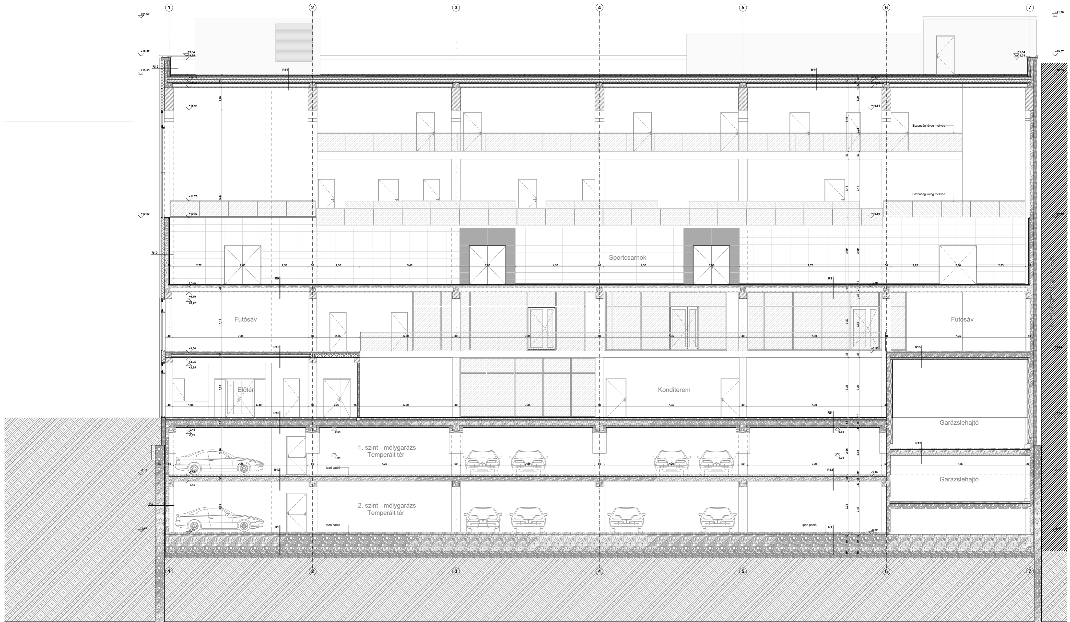
A-A metszet M= 1:100
