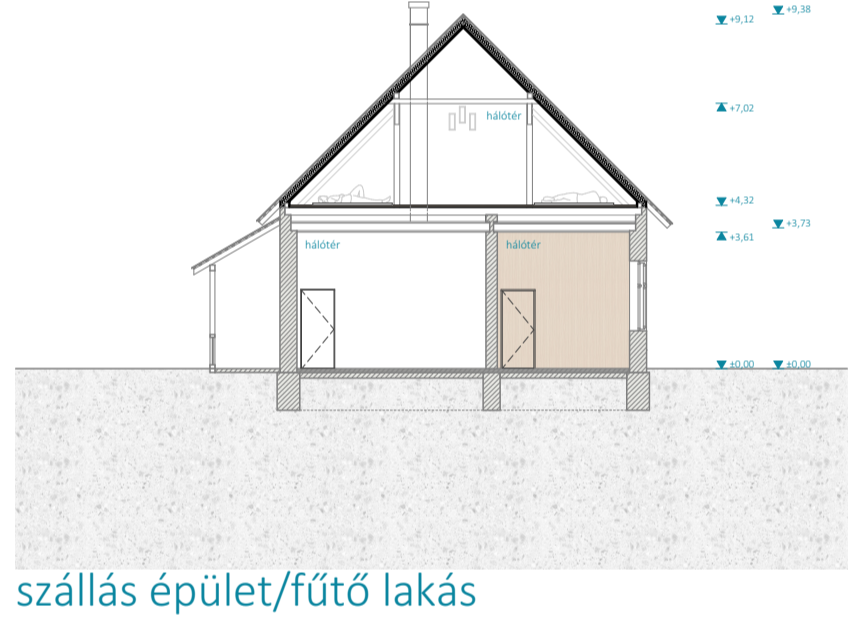
szállás épület/fűtő lakás tetőtér
