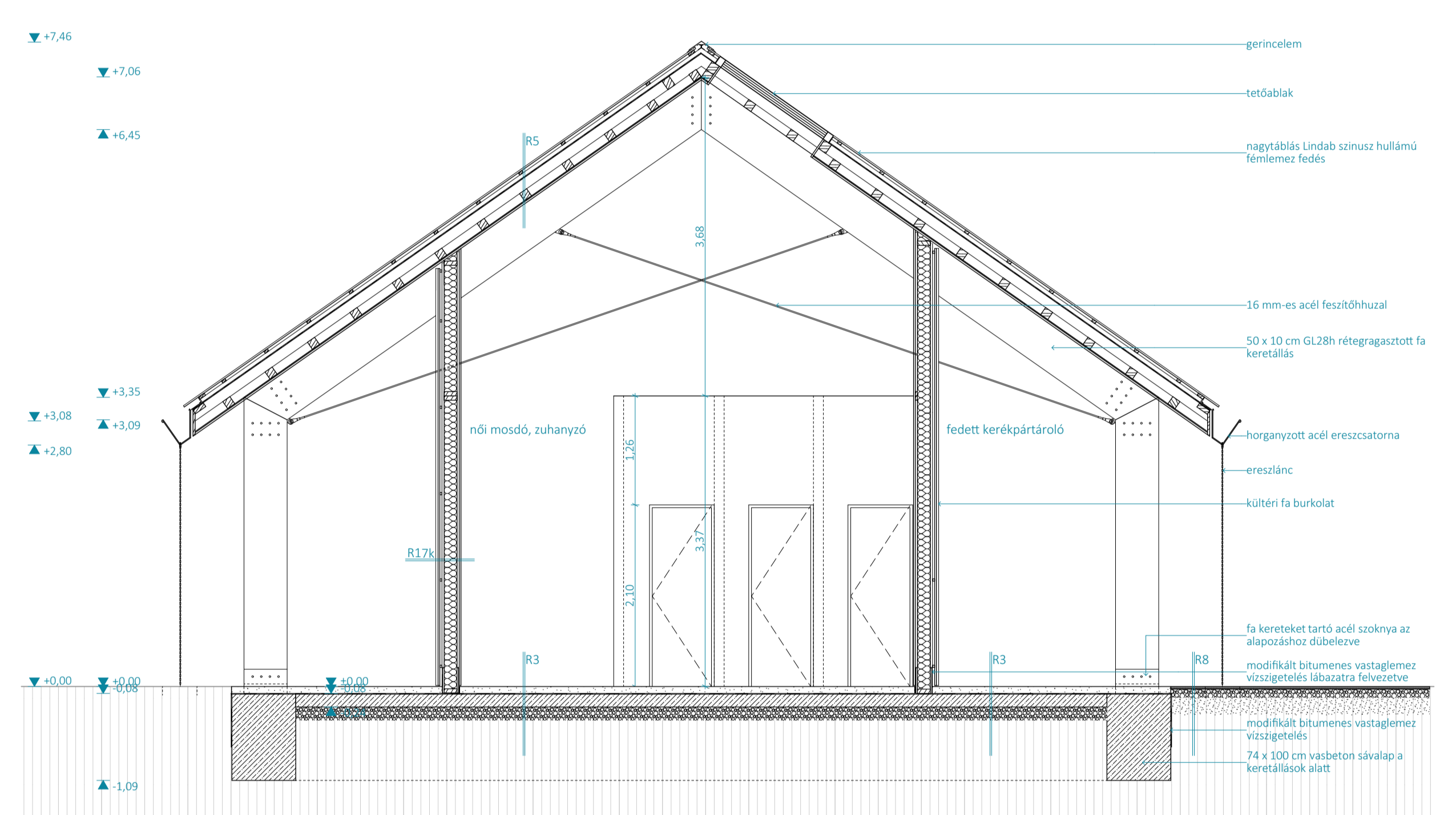
KEMPING ÉPÜLET M3 KERESZTMETSZET M=1:50
