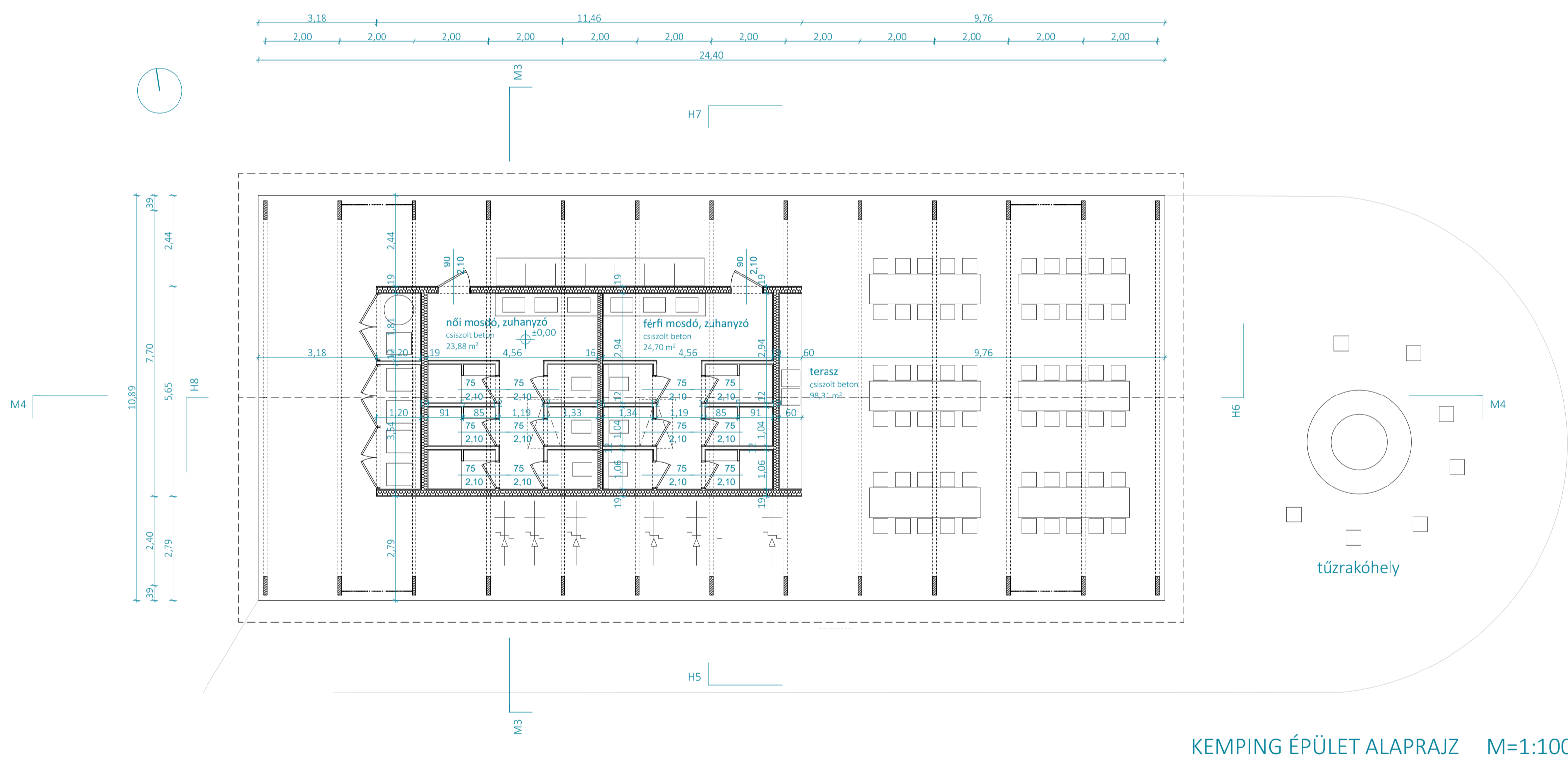
KEMPING ÉPÜLET ALAPRAJZ M=1:100
